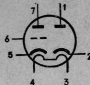
Miniatur B7G
